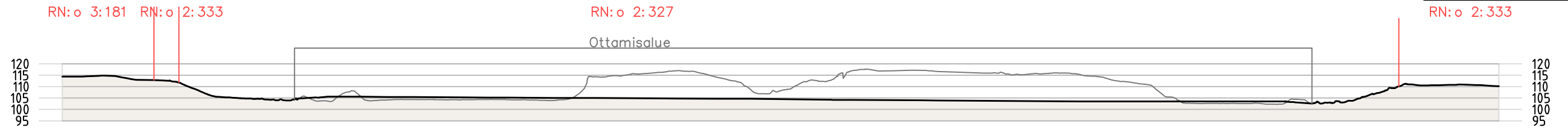
POIKKILEIKKAUS 5-5 1:2000/1:2000
