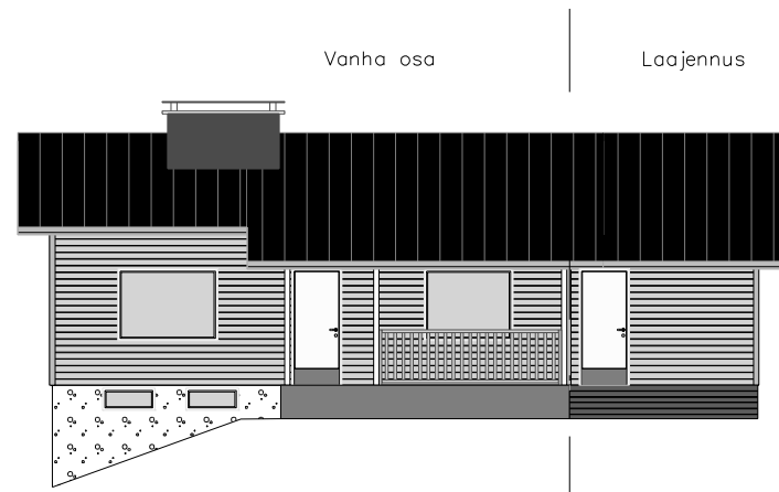
JULKISIVU Pohjoiseen
