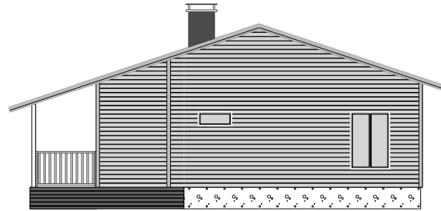
JULKISIVU Länteen
