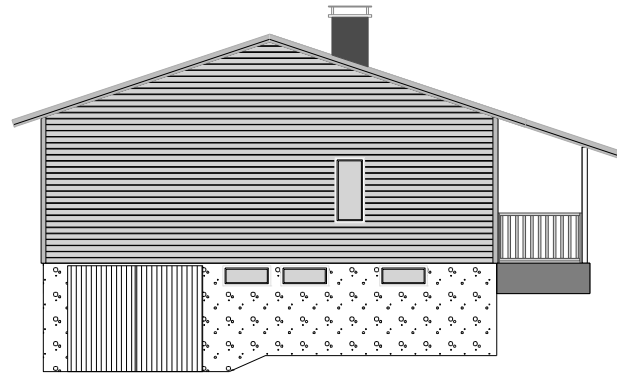
JULKISIVU Itään
