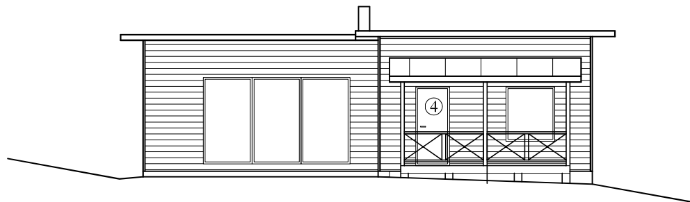
Julkisivu kaakkoon
