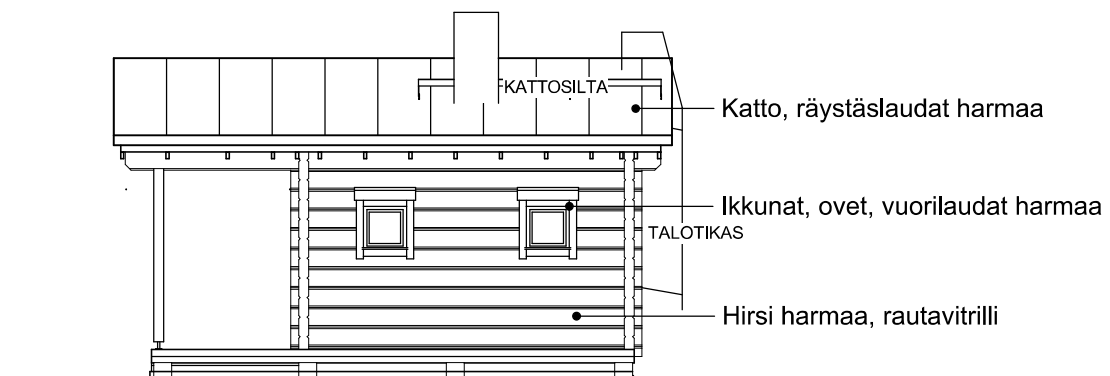
JULKISIVU POHJOISEEN
