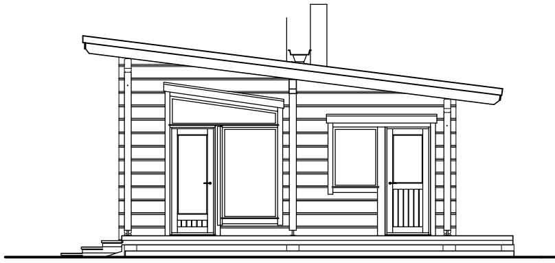
JULKISIVU ITÄÄN
